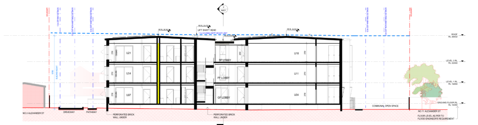
1 LONG SECTION 1 : 100
