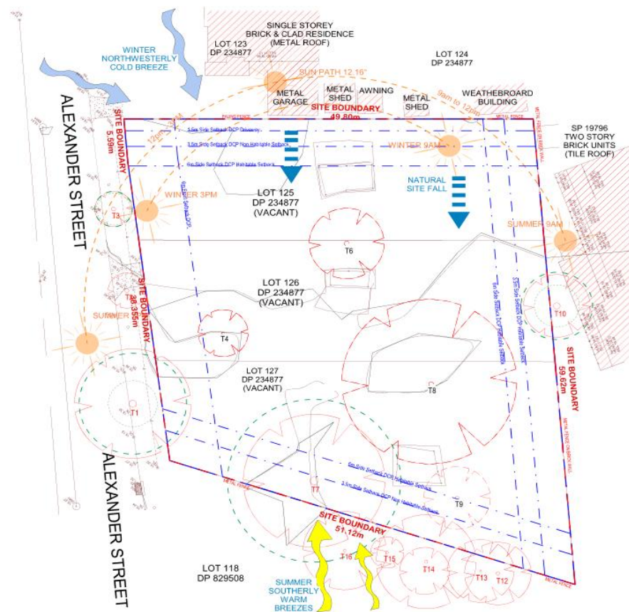
1 SITE ANALYSIS 1 : 200
